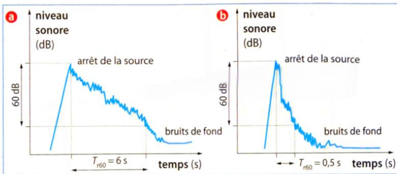
Fig. 1 Temps de réverbération pour : a une salle très réverbérante ; b une salle peu réverbérante.
